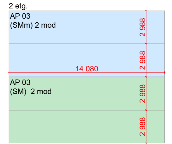
Module positioning 1:200
