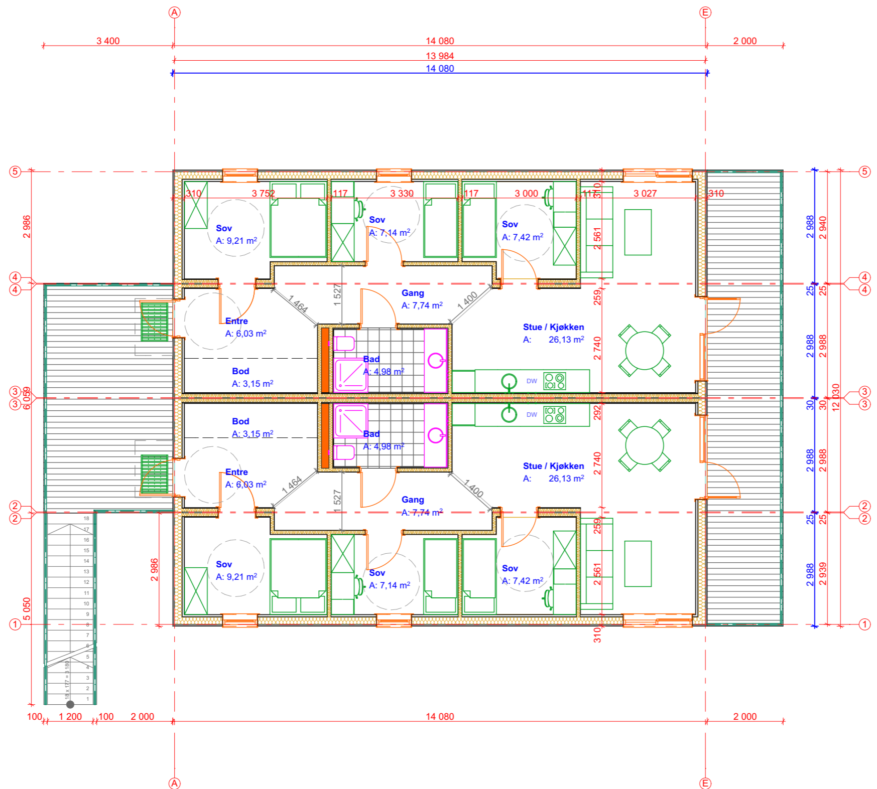
2 etg. 1:100
